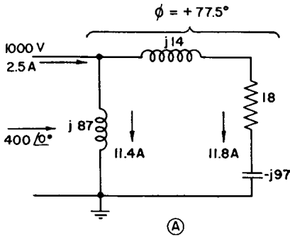
FIG. 2.26. Network A.
