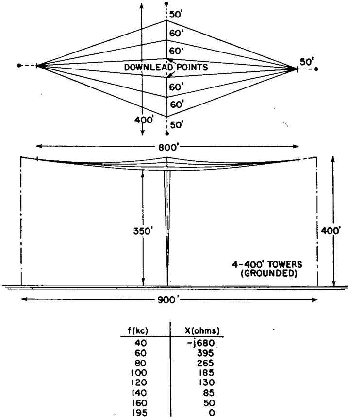
FIG. 1.32. Diamond antenna.
