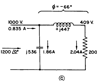
FIG. 2.28. Network C.
